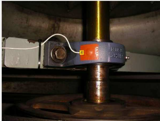
軸承測溫點
