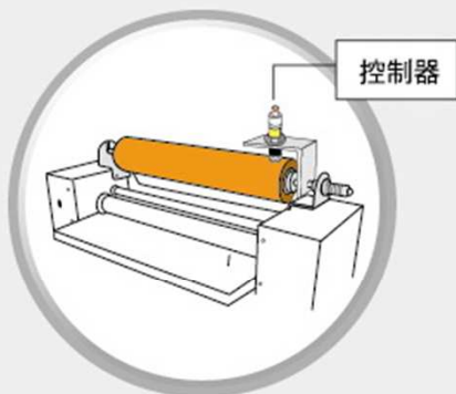
加熱滾輪
